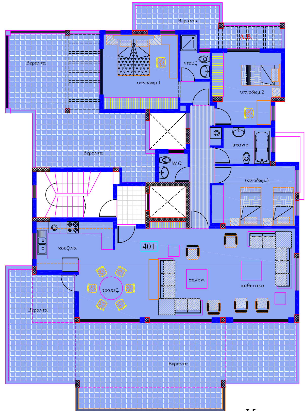
Κατοψη 4ου Οροφου
