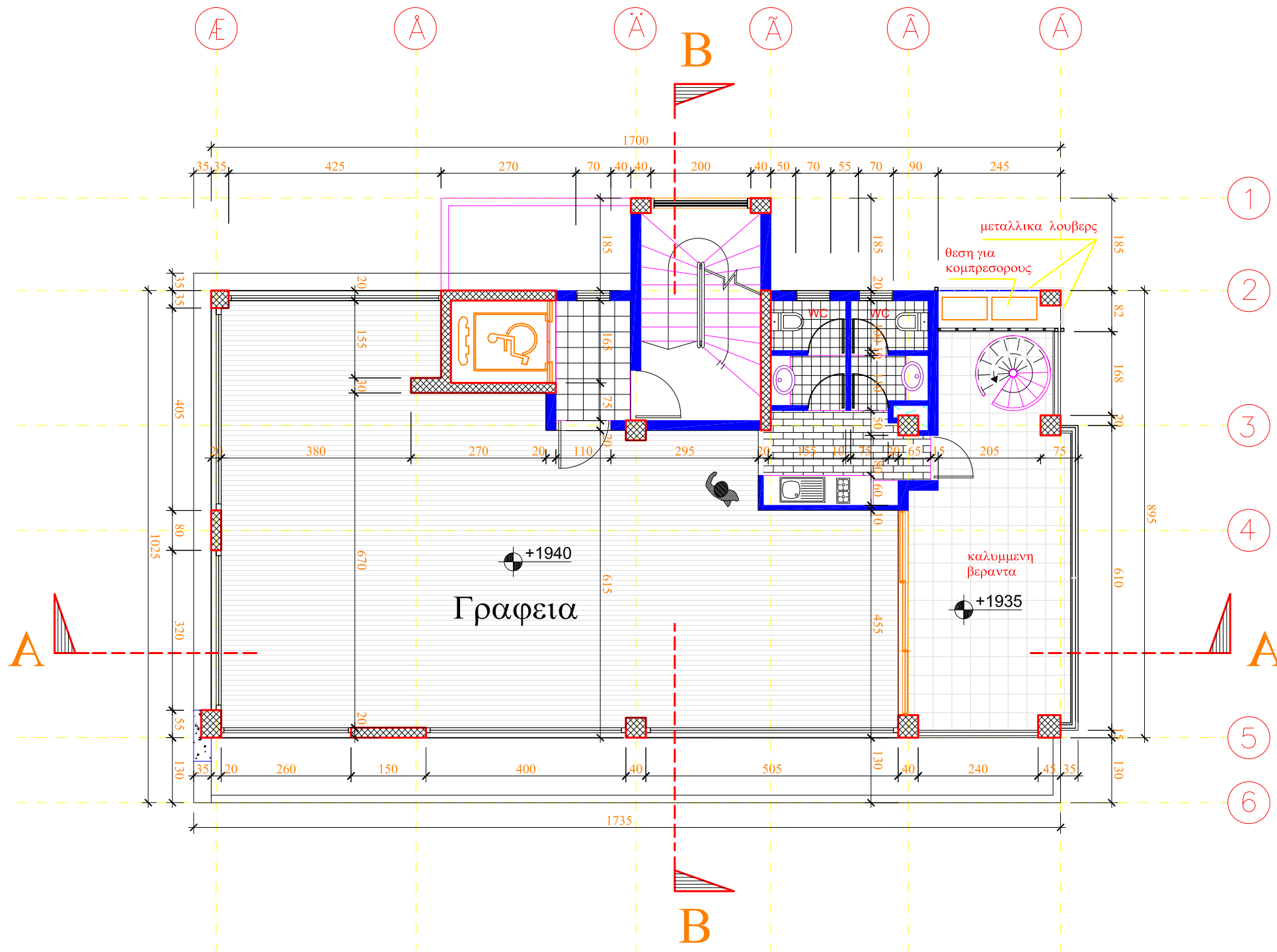
ΚΑΤΟΨΗ 5ου ΟΡΟΦΟΥ
